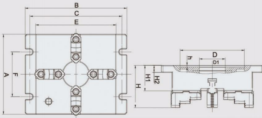
尺寸、性能参数 Dimension characteristic parameters
