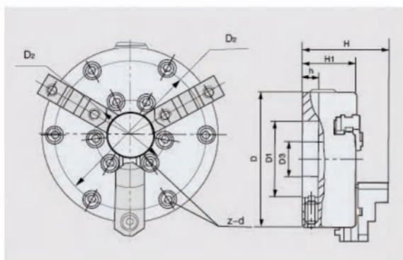
尺寸、性能参数 Dimension characteristic parameters
