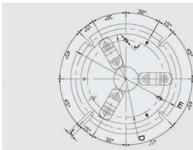
尺寸、性能参数 Dimension characteristic parameters
