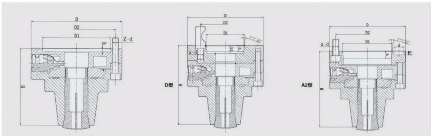
尺寸、性能参数 Dimension characteristic parameters
