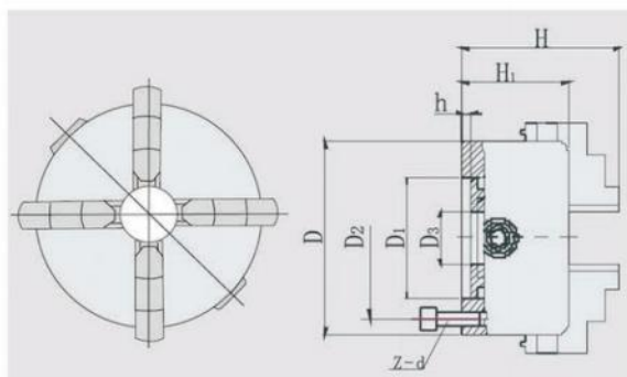
尺寸、性能参数 Dimension characteristic parameters
