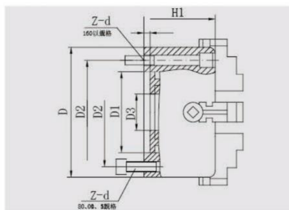
K72——四爪单动卡盘(美标)
