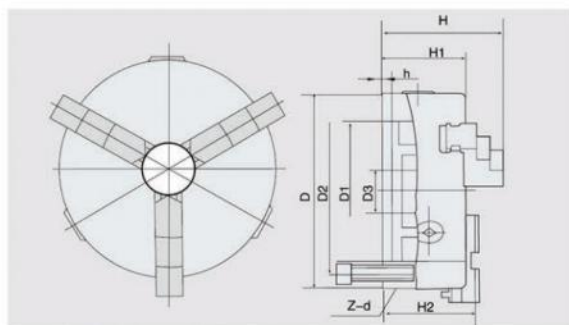
尺寸参数 Dimension parameters
